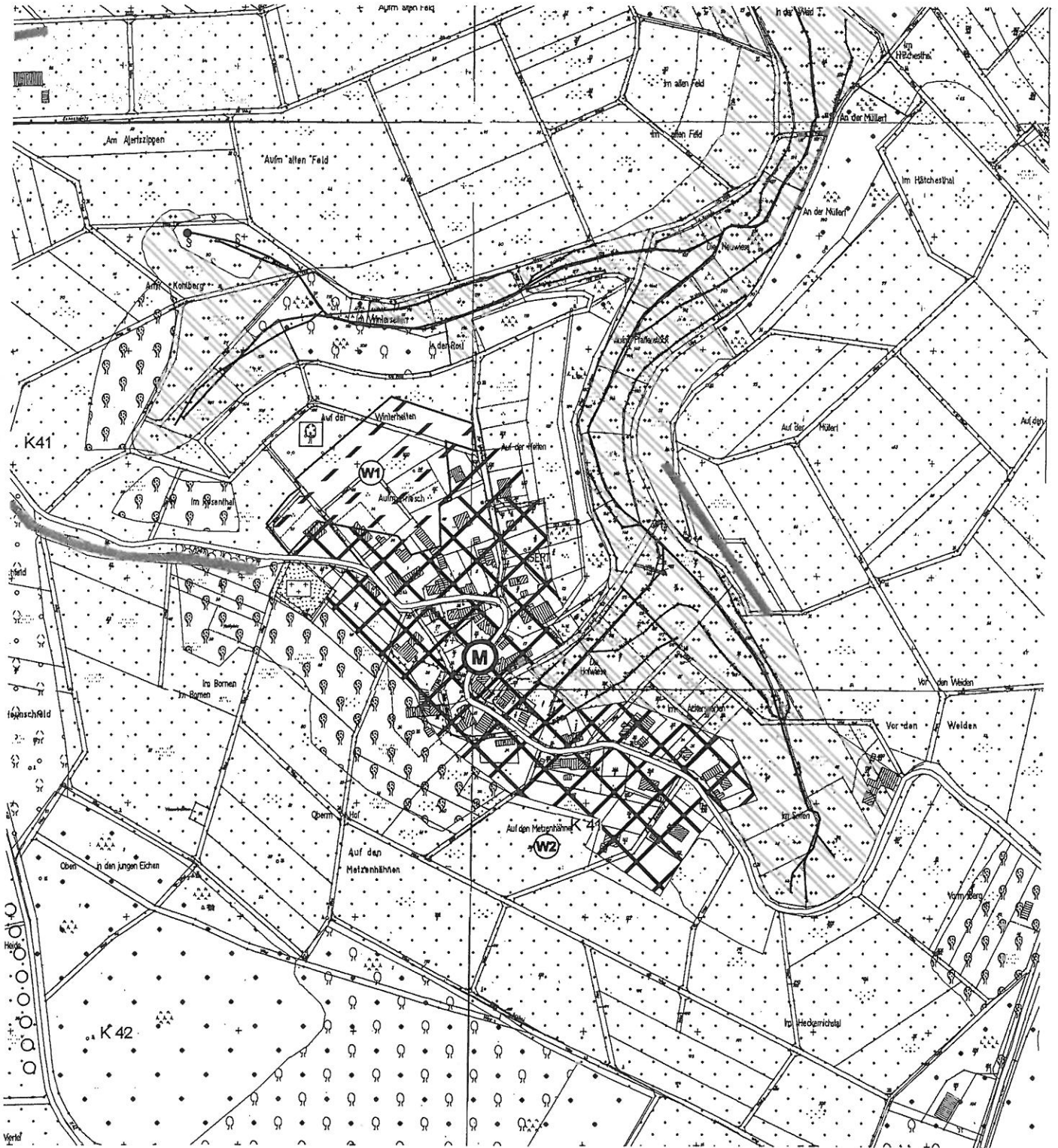
Stadt-Land-plus Flächennutzungsplan VG Altenkirchen Ortsgemeinde Isert Maßstab 1:5.000
